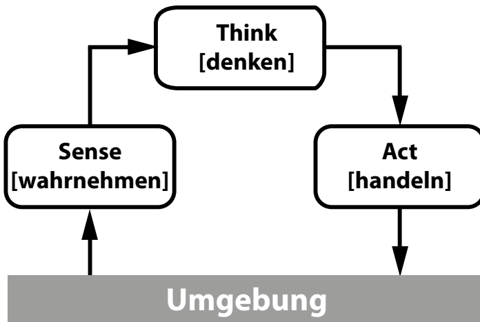
Abbildung 6: Das Sense-Think-Act-Modell.
